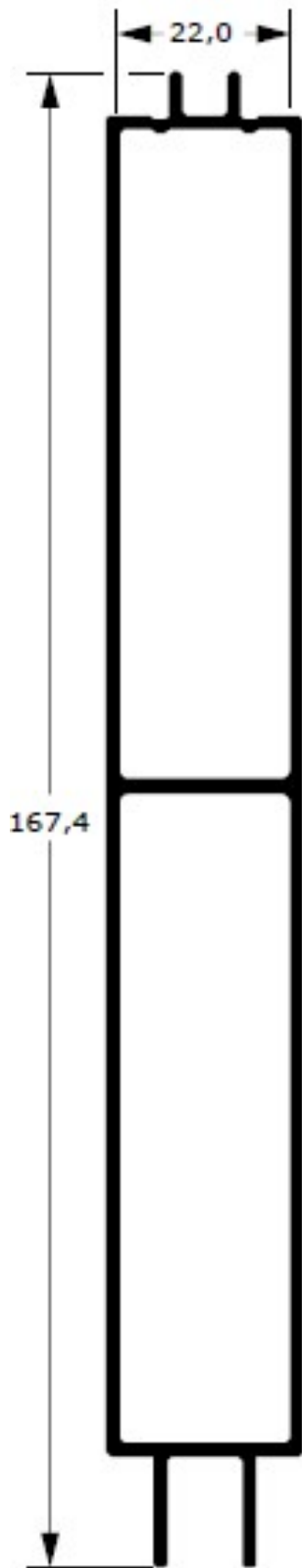
78-1740 1,804 kg/m
