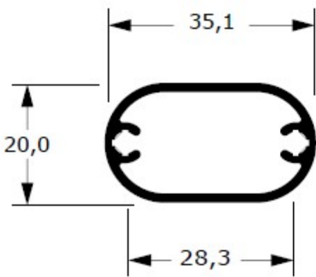
78-366 0,427 kg/m
