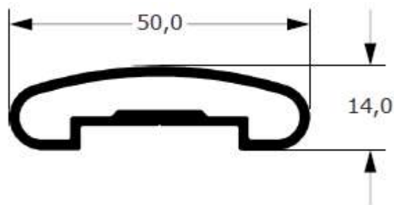
CG-003 0,544 kg/m
