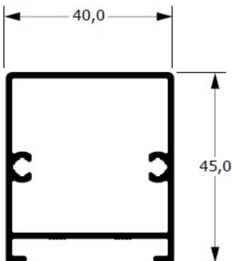
78-366 0,427 kg/m
