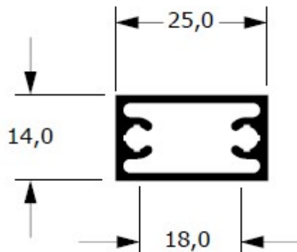
CG-021 0,349 kg/m
