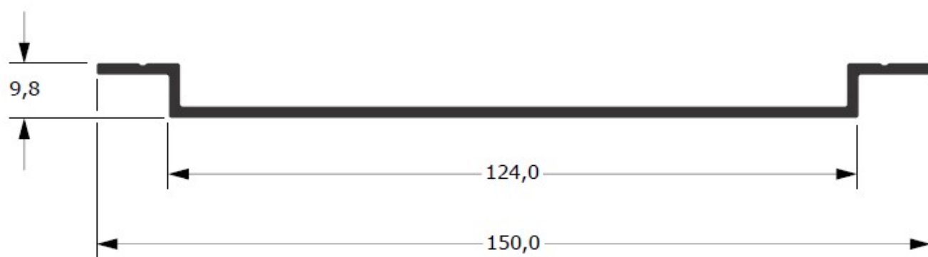
31-085 0,894 kg/m
