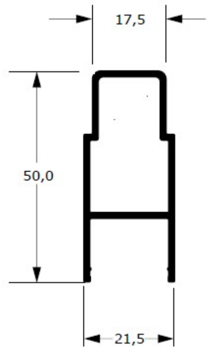
78-2226 0,555 kg/m
