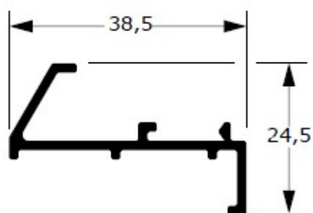
DS-005 0,325 kg/m
