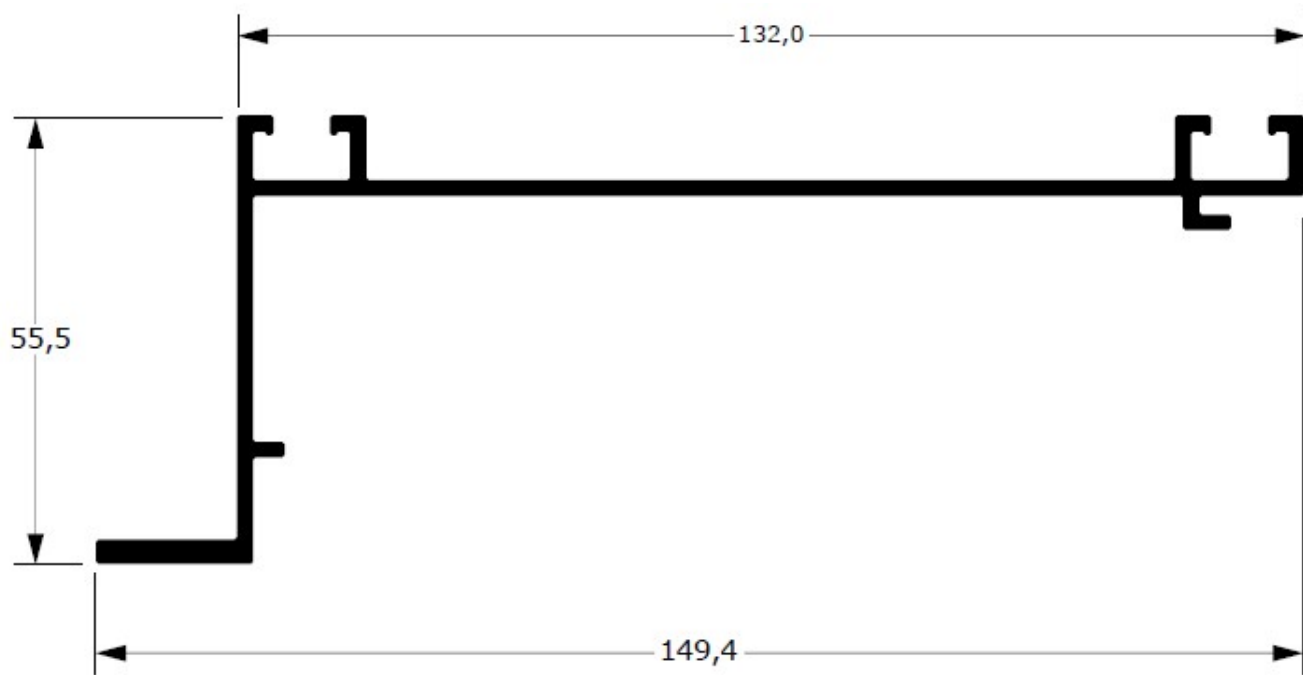
29-160 1,398 kg/m
