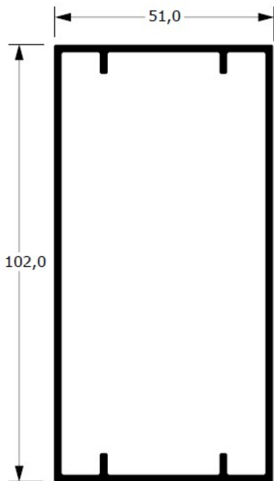
78-719 1,555 kg/m
