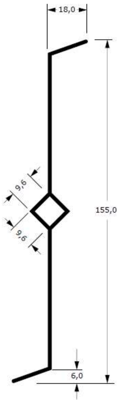
DC-006 0,835 kg/m
