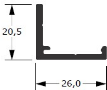
29-317 0,290 kg/m
