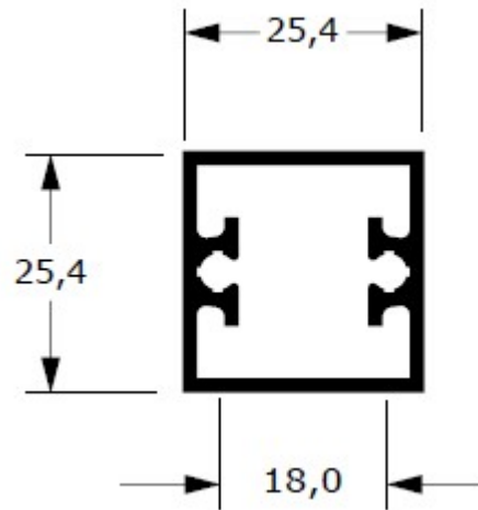
D-080 0,524 kg/m
