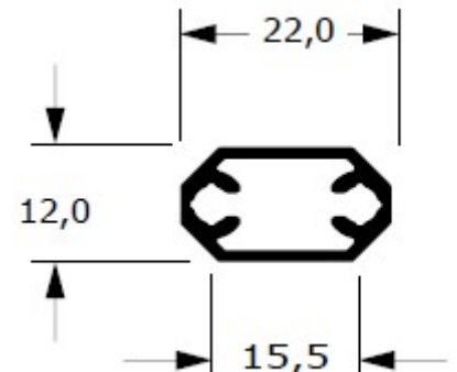
CG-022 0,256 kg/m
