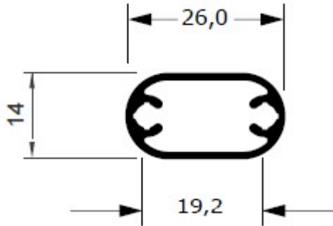
78-1017 0,286 kg/m
