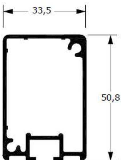
CG-077 0,859 kg/m
