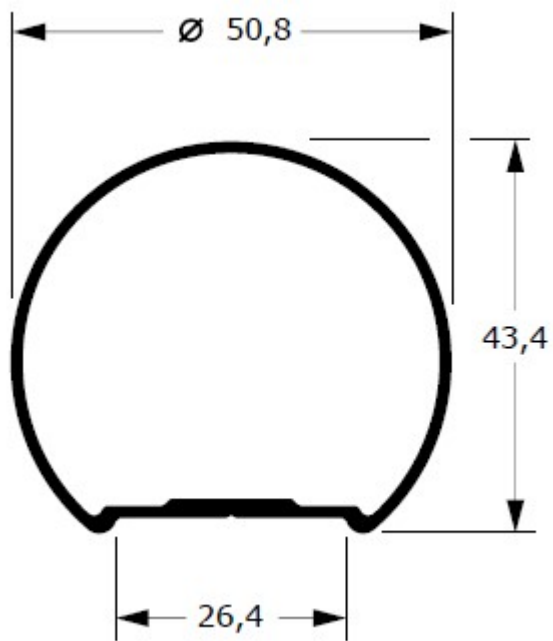
CG-300 0,664 kg/m
