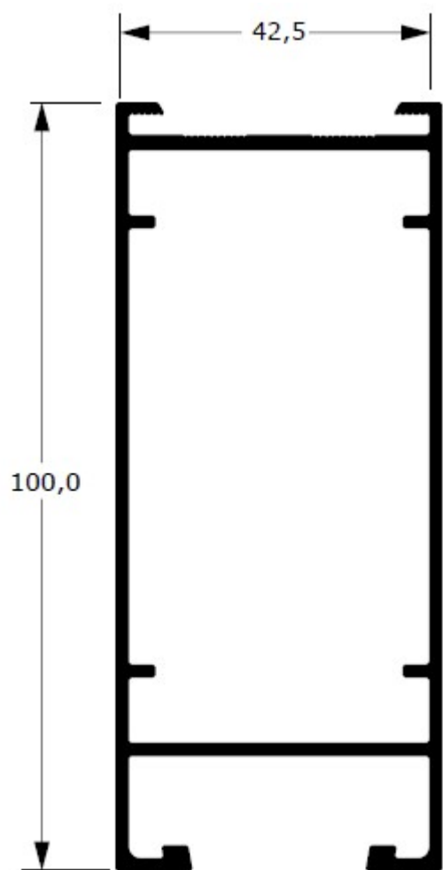
78-1730 1,510 kg/m
