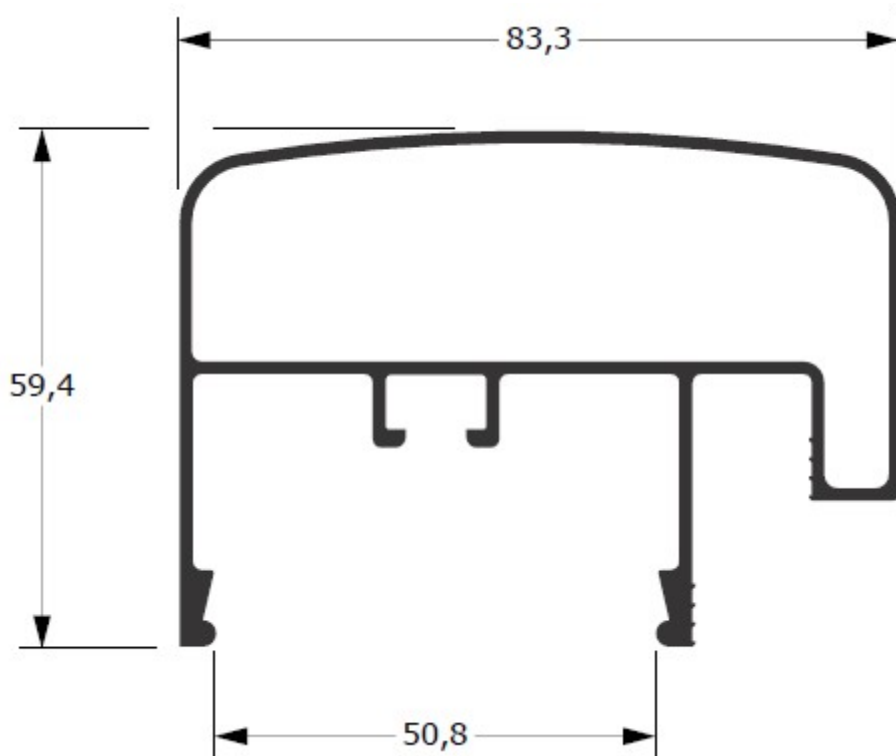
CG-083 1,345 kg/m
