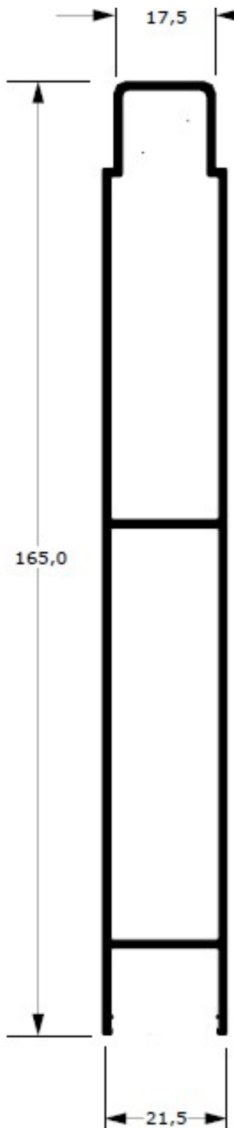
79-060 1,464 kg/m
