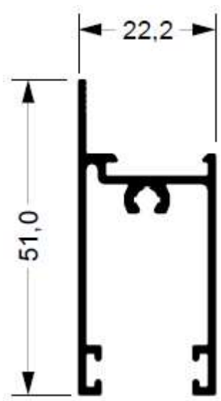
SU-053 0,542 kg/m
