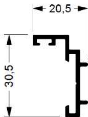
25-548 0,283 kg/m
