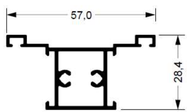
SU-086 0,589 kg/m
