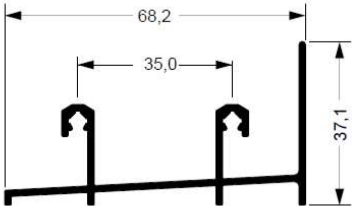
SU-228 0,791 kg/m
