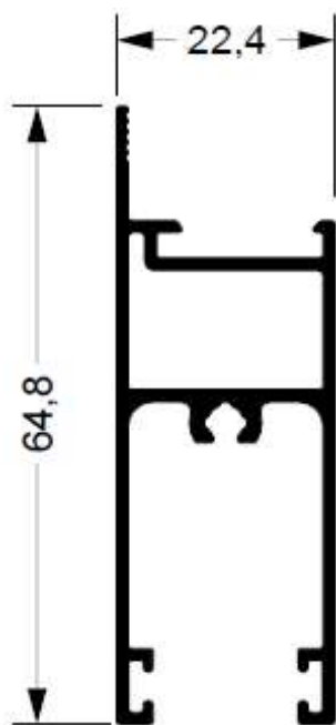
SU-246 0,645 kg/m
