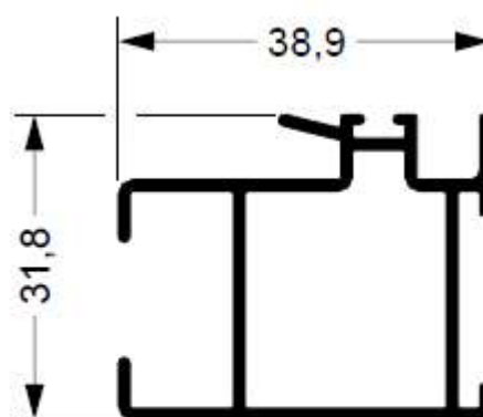
SU-057 0,632 kg/m
