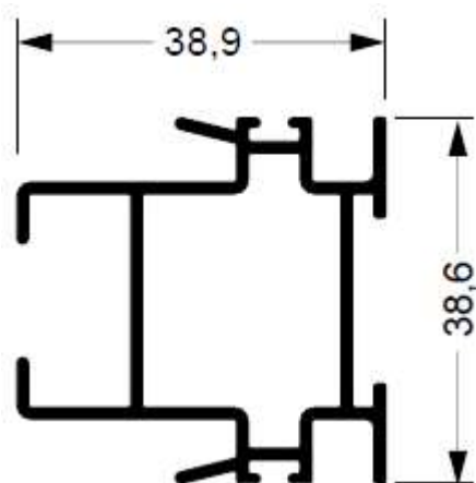
SU-056 0,538 kg/m
