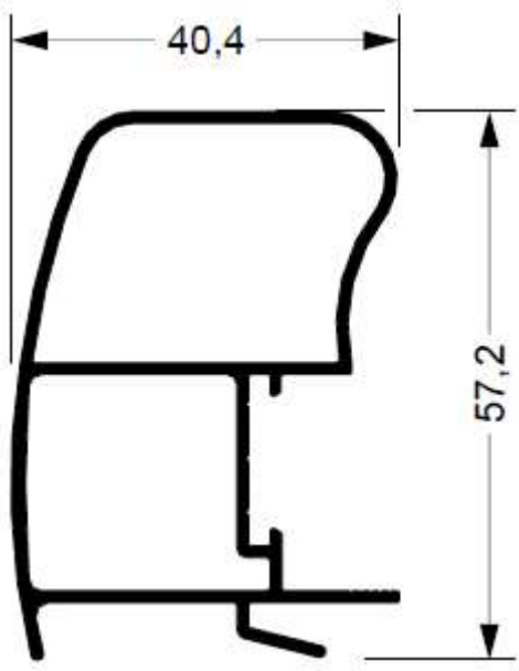
88-504 0,757 kg/m
