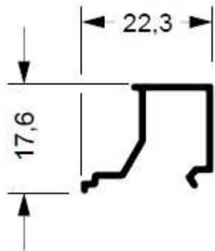
SU-103 0,104 kg/m
