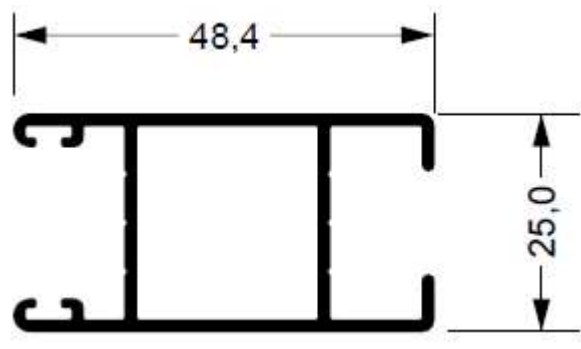
88-783 0,565 kg/m
