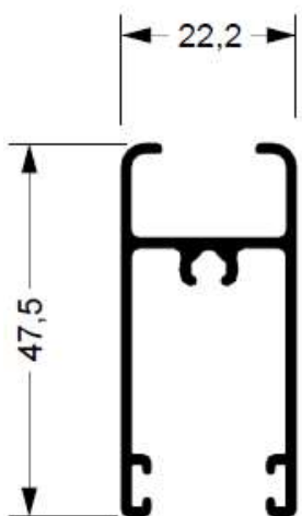
SU-186 0,496 kg/m
