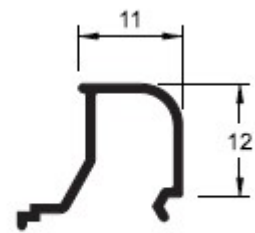
AF-018 0,104 kg/m
