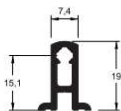
SU-017 0,233 kg/m
