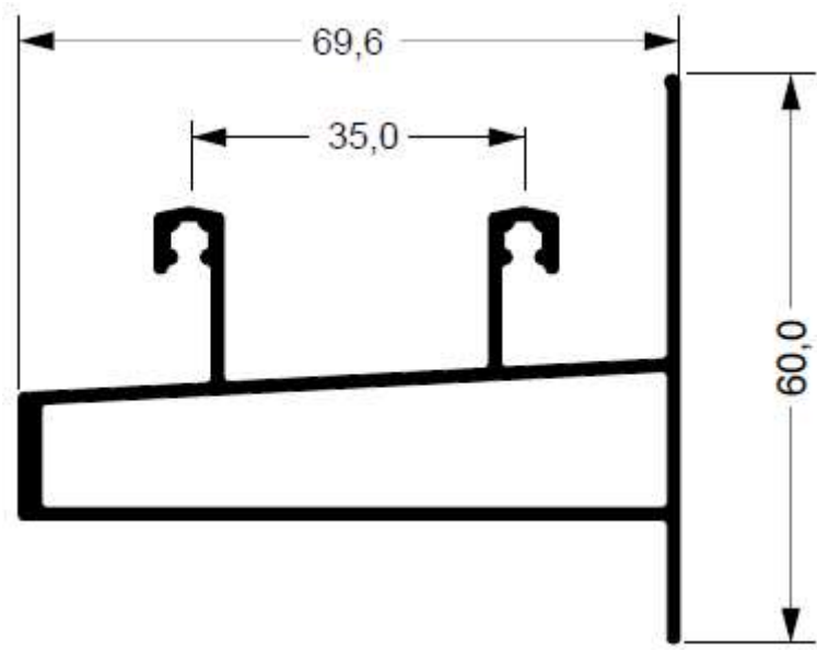
SU-006 0,999 kg/m
