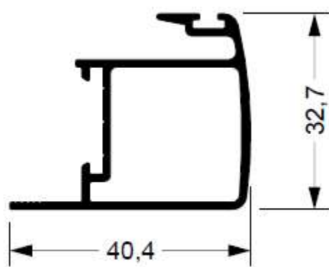
88-502 0,490 kg/m
