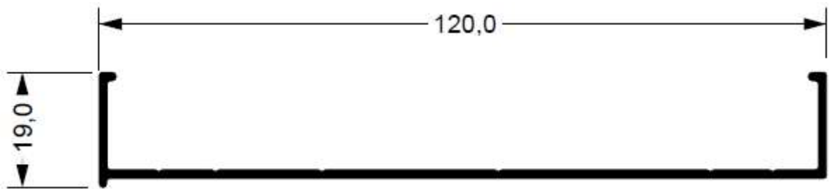
88-513 1,075 kg/m
