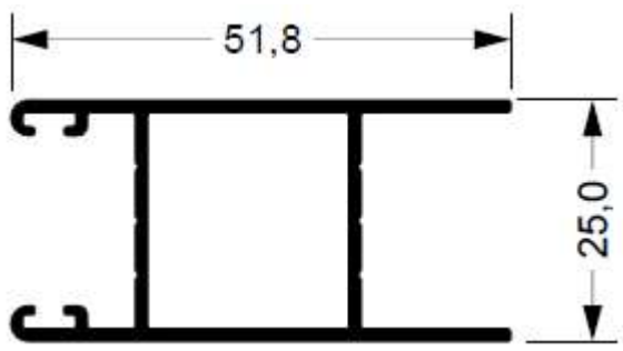
88-784 0,555 kg/m
