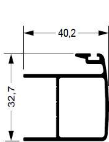
88-785 0,500 kg/m
