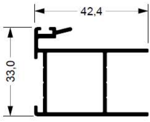
SU-070 0,559 kg/m
