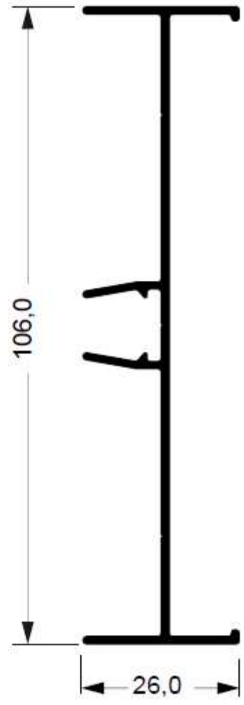
SU-014 0,671 kg/m
