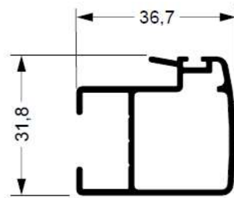
88-787 0,513 kg/m
