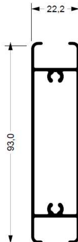
88-790 0,871 kg/m
