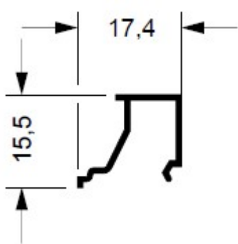
SU-102 0,110 kg/m
