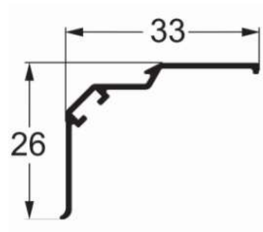
SU-276 0,170 kg/m
