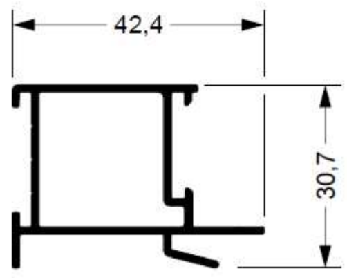
SU-040 0,482 kg/m
