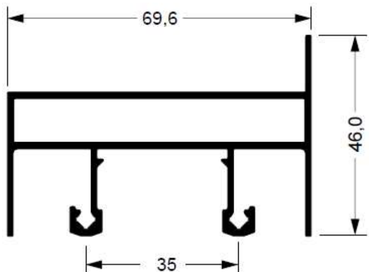
SU-005 1,106 kg/m
