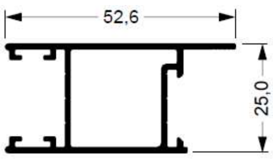
SU-039 0,554 kg/m
