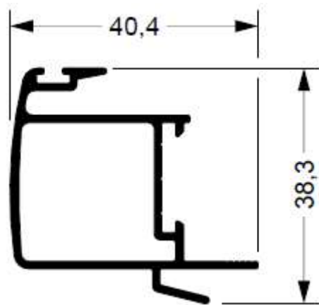
88-503 0,523 kg/m
