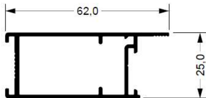
SU-111 0,634 kg/m
