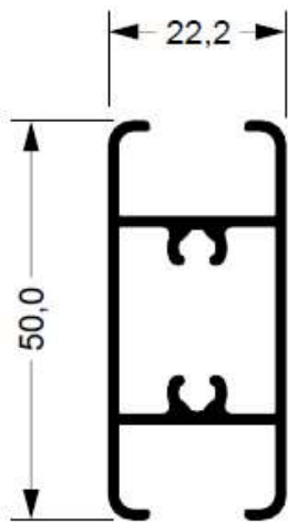
SU-188 0,586 kg/m
