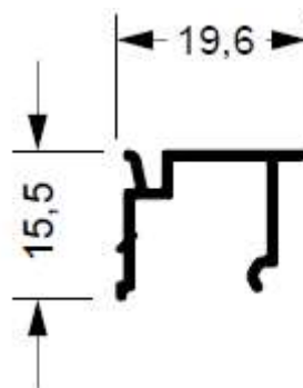
SU-203 0,107 kg/m
