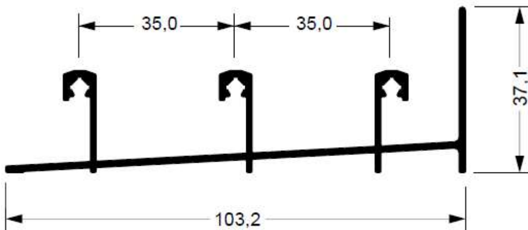
SU-230 0,976 kg/m
