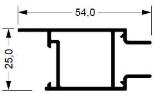
SU-192 0,554 kg/m
