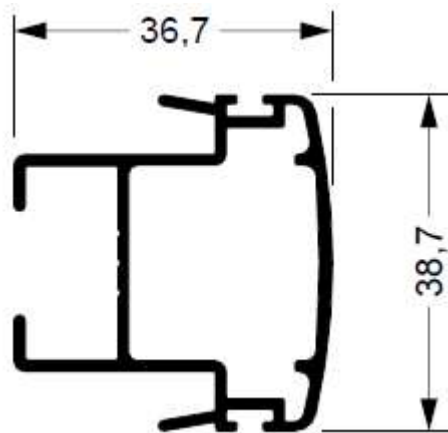
88-788 0,599 kg/m
