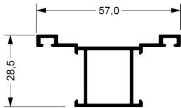
SU-085 0,506 kg/m
