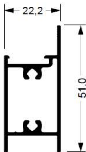
SU-110 0,554 kg/m
