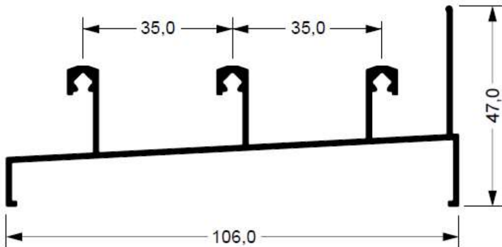
SU-011 0,960 kg/m
