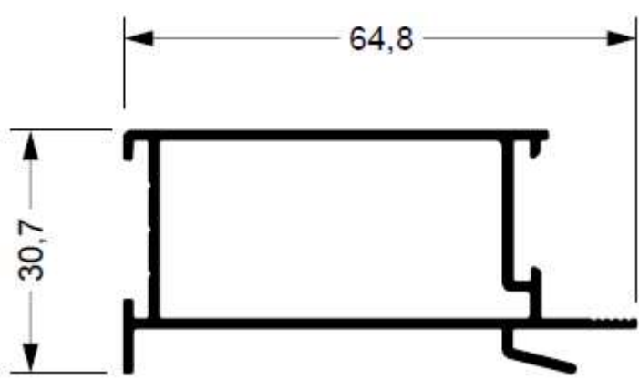
SU-243 0,636 kg/m
