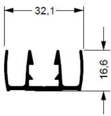
88-507 0,383 kg/m
