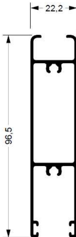
SU-226 0,945 kg/m
