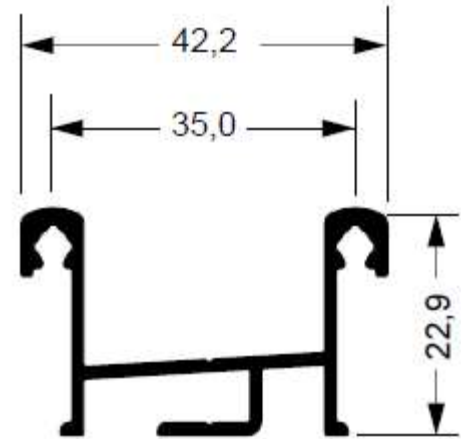
SU-272 0,430 kg/m
