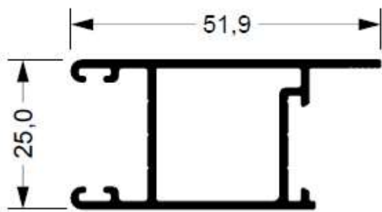
88-500 0,542 kg/m
