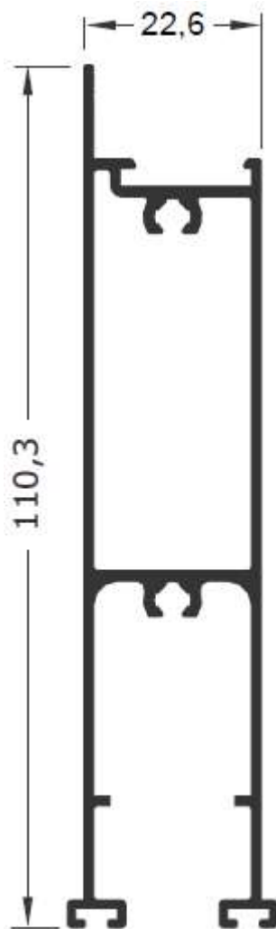
SU-247 1,015 kg/m
