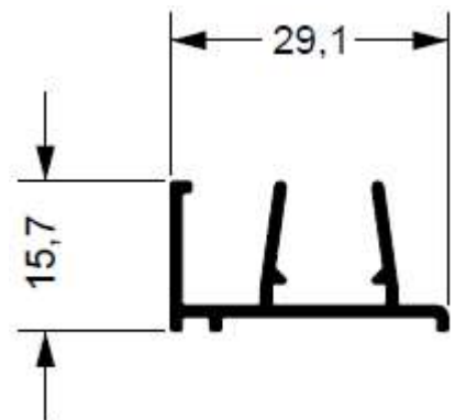
SU-008 0,245 kg/m
