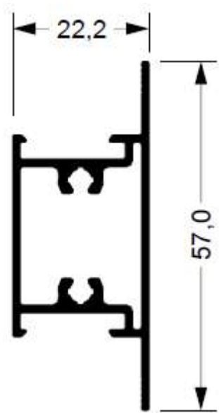
SU-227 0,574 kg/m
