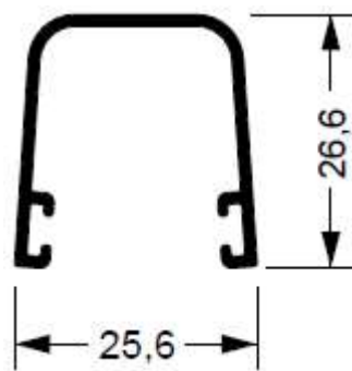
SU-107 0,269 kg/m
