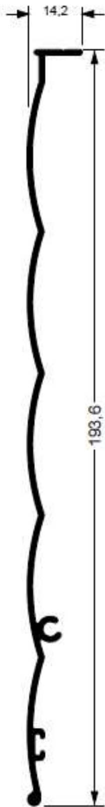
88-518 0,885 kg/m
