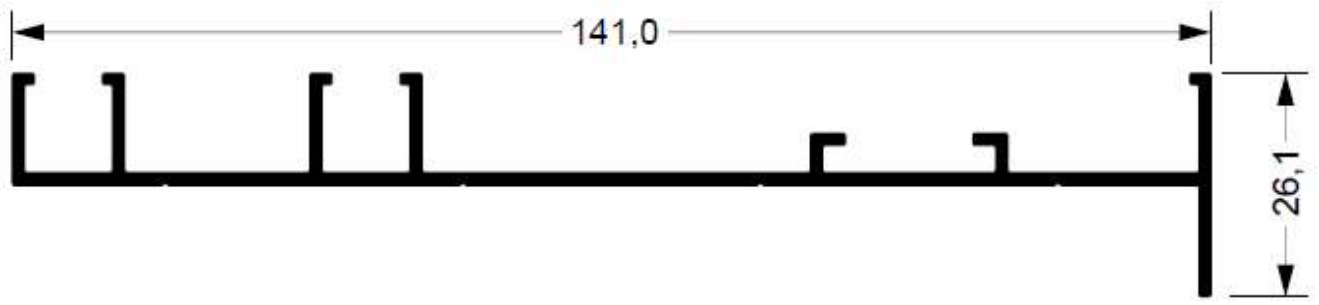
SU-123 0,917 kg/m
