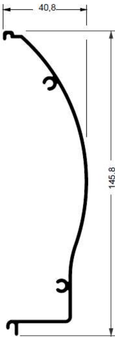
88-515 0,857 kg/m
