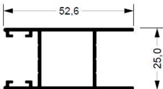
SU-068 0,574 kg/m
