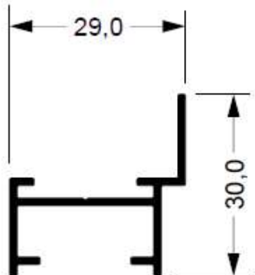
SU-071 0,279 kg/m
