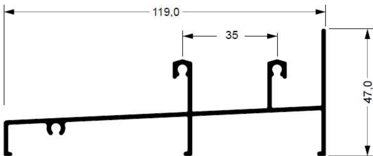
88-510 1,085 kg/m
