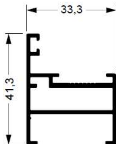
SU-279 0,565 kg/m
