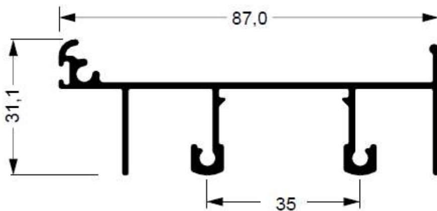
88-509 0,843 kg/m
