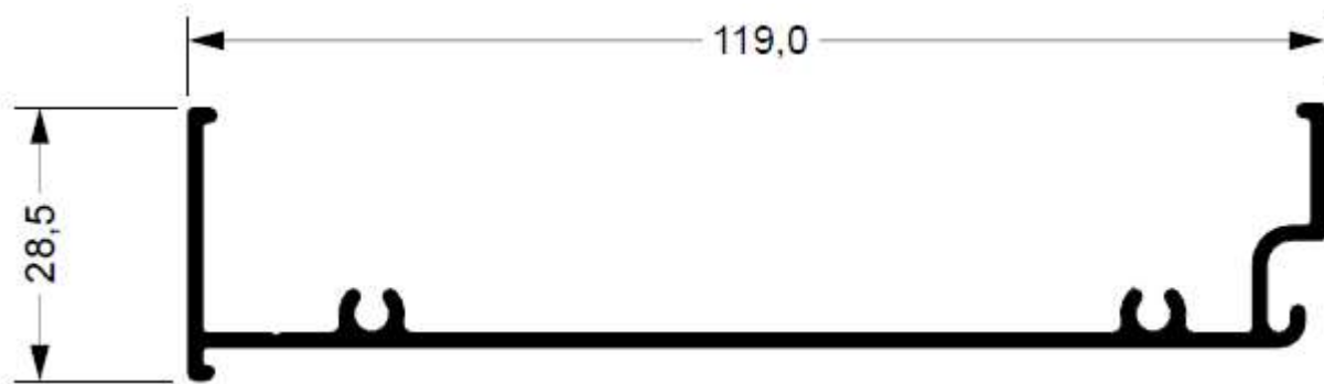
88-508 0,810 kg/m
