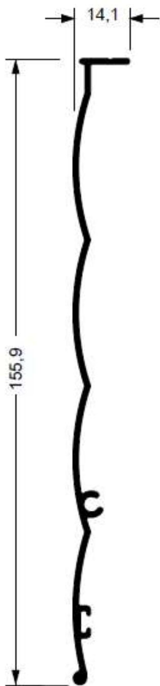
88-516 0,724 kg/m
