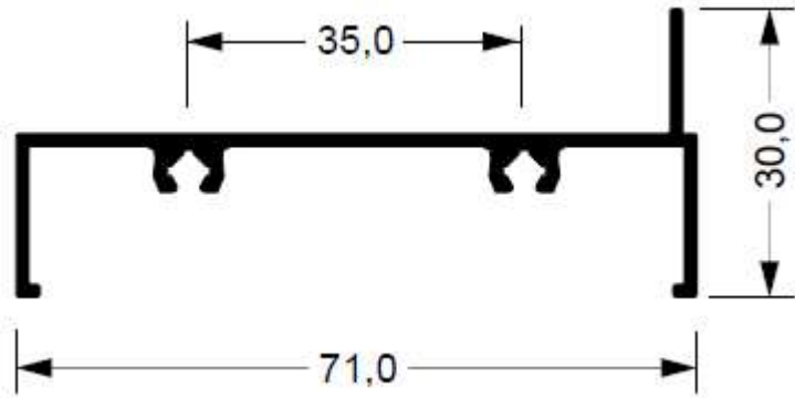
SU-004 0,526 kg/m
