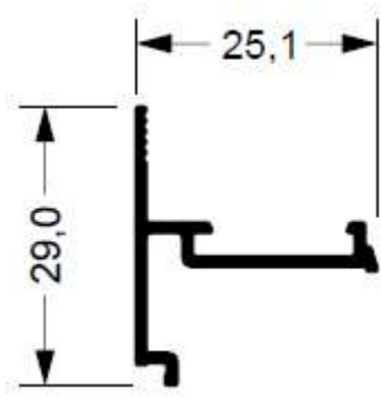
SU-292 0,214 kg/m
