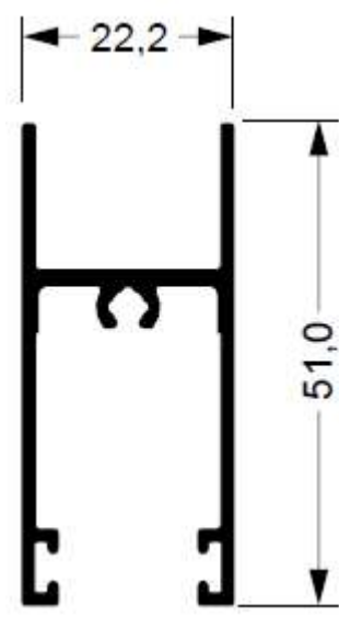
SU-187 0,534 kg/m
