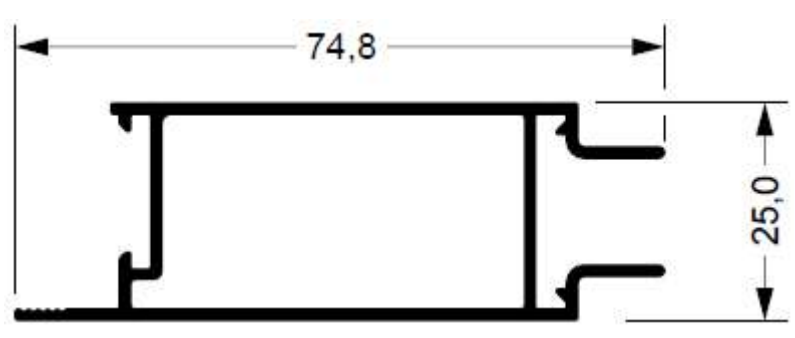
SU-244 0,699 kg/m
