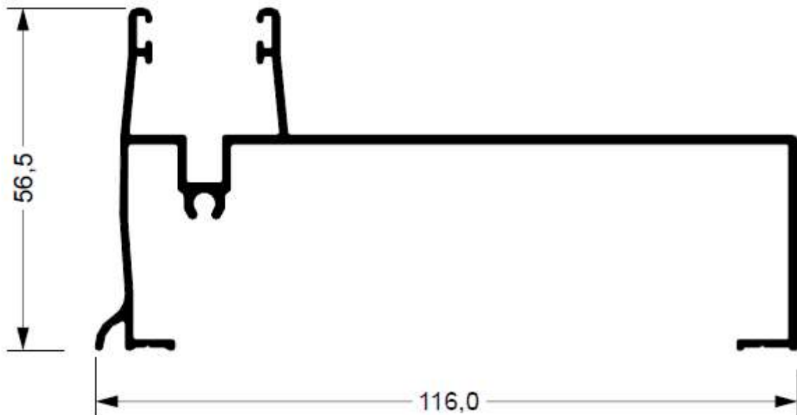
88-513 1,075 kg/m
