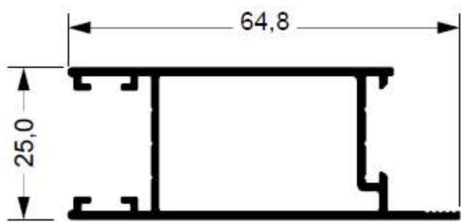
SU-245 0,636 kg/m
