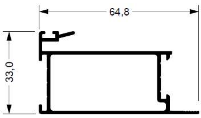
SU-242 0,674 kg/m
