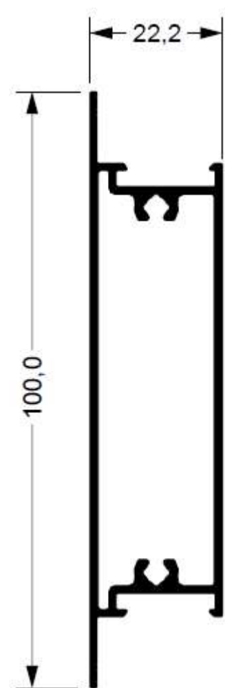
SU-050 0,926 kg/m
