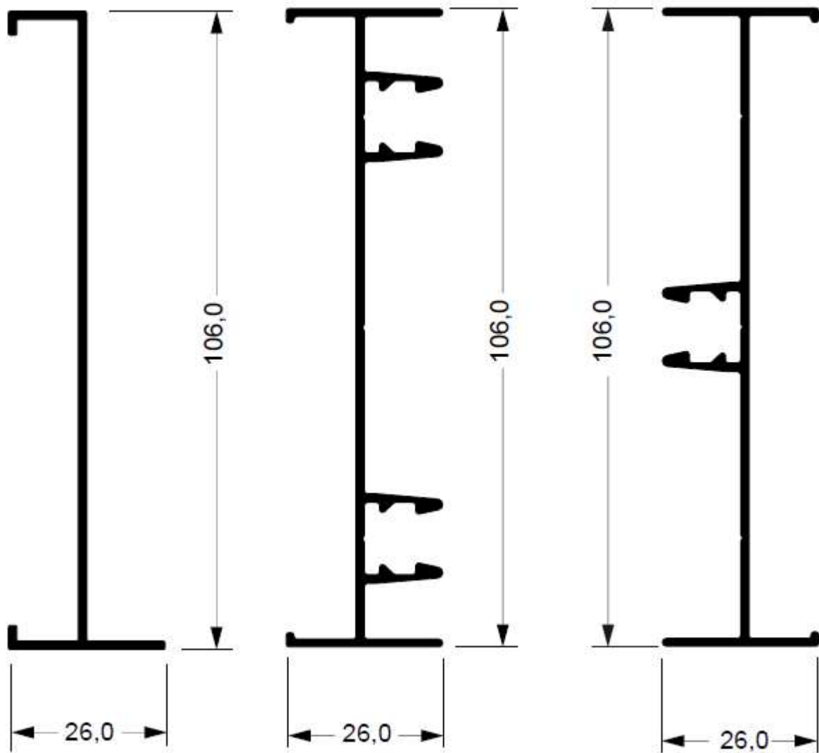
SU-012 0,559 kg/m
