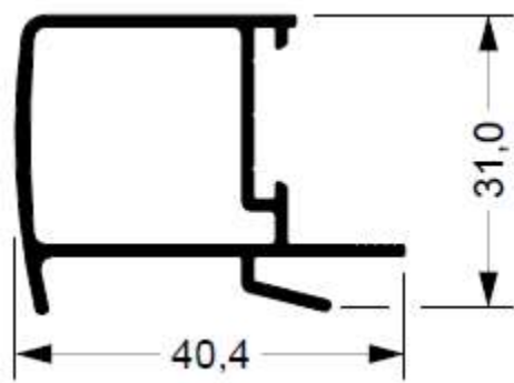
88-501 0,458 kg/m
