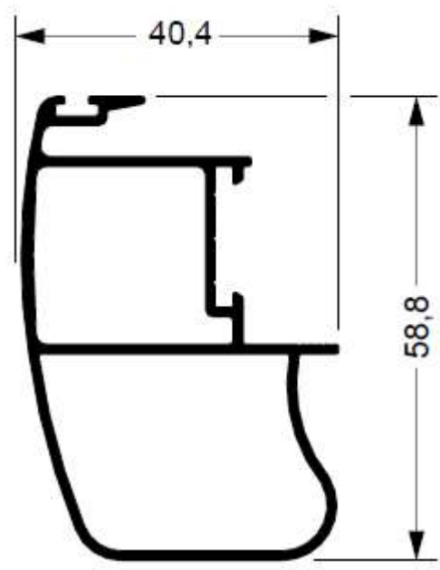
88-505 0,745 kg/m
