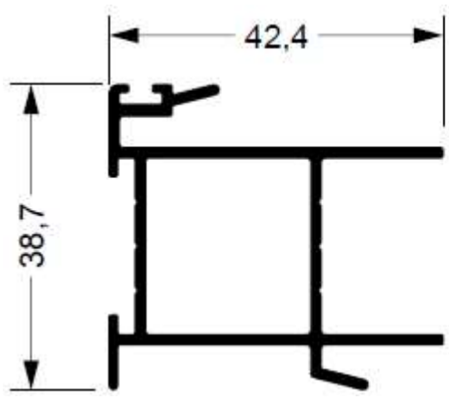
SU-069 0,613 kg/m
