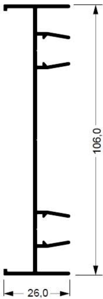
SU-013 0,767 kg/m
